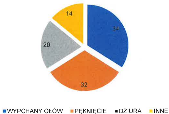
Wykres nr 5 Awarie według charakterystyki uszkodzenia w 2024 r.
