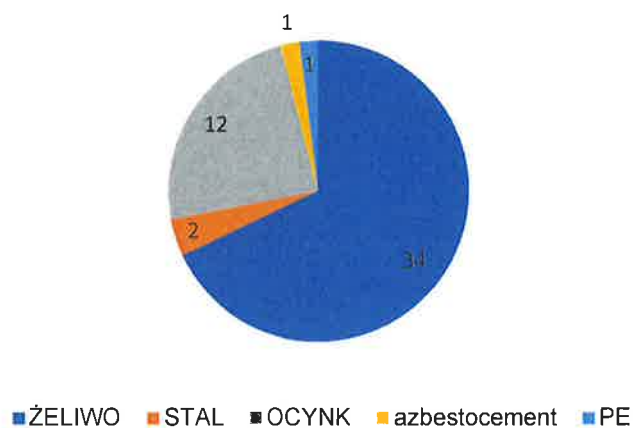
Wykres nr 4 Zestawienie ilości awarii na sieci i przyłączach wg materiału w 2024 r.
