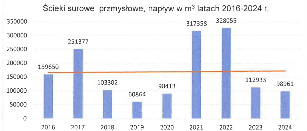
Wykres nr 11 Napływ ścieków przemysłowych do oczyszczalni ścieków w latach 2016 - 2024 w tys. m 3 .
