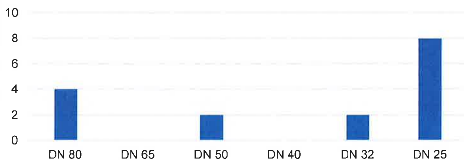
Wykres nr 3 Zestawienie ilości awarii na przyłączach wg średnic w 2024 r.
