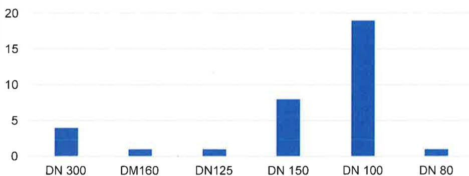
Wykres nr 2 Zestawienie ilości awarii na sieci wg średnic w 2024 r.
